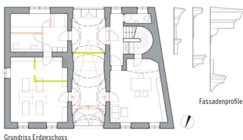
Grundriss Erdgeschoss
